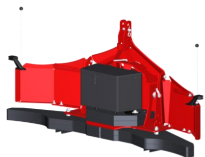
Werkzeugbox mit max. Ballastierung (2x 90kg und 2x 250kg Gewichtsplatten)
