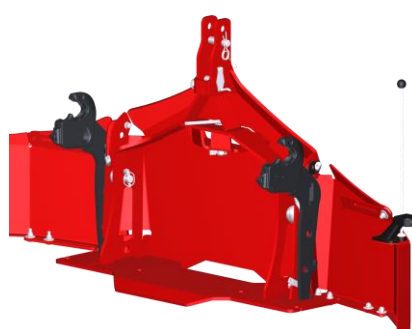
Fanghaken (in Transportstellung)
